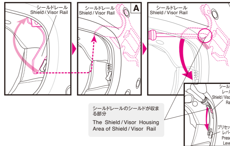
プリセットレバー Preset Lever
