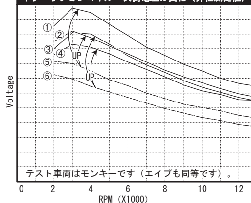
イグニッションコイル一次側電圧の変化（弊社測定値）
