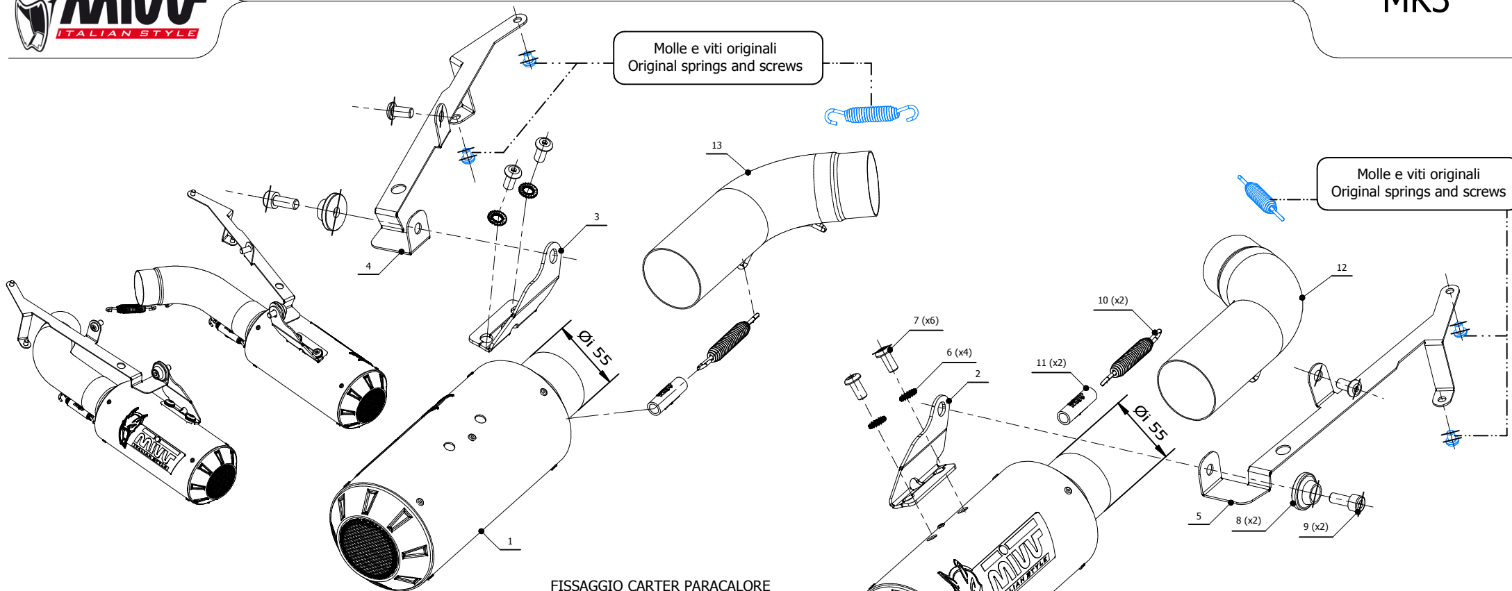
FISSAGGIO CARTER PARACALORE HEAT SHIELD FIXING
