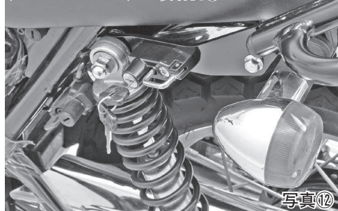
汎用 ヘルメットホルダーセット（ブラック） （EH507HANB1）の装着例①
