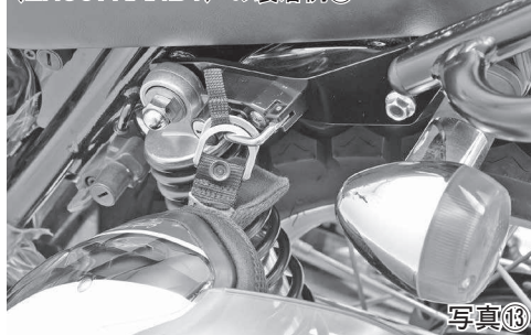
汎用 ヘルメットホルダーセット（ブラック） （EH507HANB1）の装着例②
