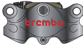
Φ34 ニッケルコーティング 品番 120.A441.40
